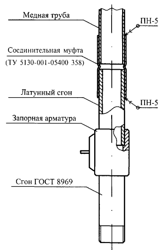
Рисунок 6 — Присоединение запорной арматуры к медному газопроводу
