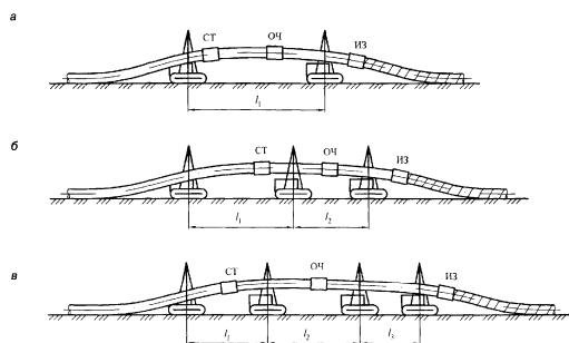
Рисунок 19 — Схема расстановки трубоукладчиков для укладки плети газопровода (см. таблицу 24) ОИ — установка очистки, ИЗ — изоляционная установка
