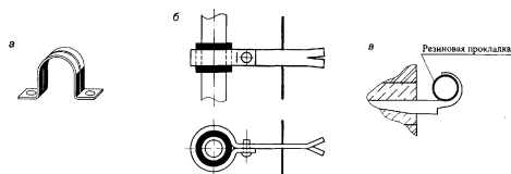
Рисунок 5 — Опоры для крепления медных газопроводов
