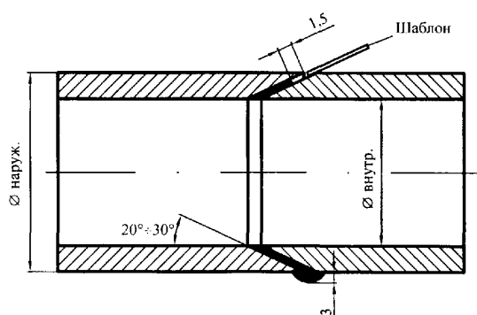
Рисунок 11 — Паяное соединение стальных труб
