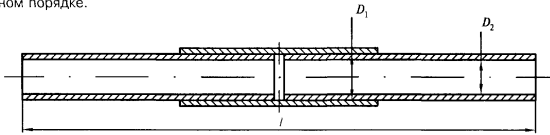
Рисунок 8 — Допускное соединение
