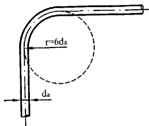
Рисунок 13 — Холодная гибка медной трубы
