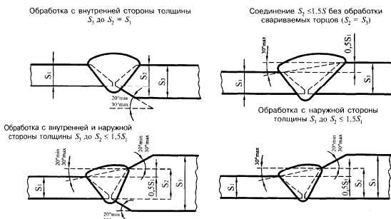
Рисунок 10 — Обработка свариваемых торцов труб
