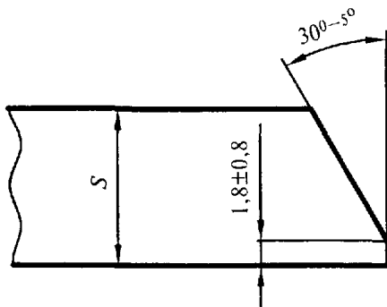
Рисунок 9 — Схема обработки кромки
