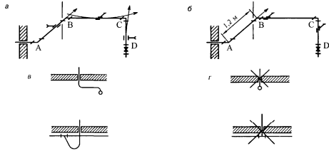
Рисунок 7 — Прокладка газопроводов с соблюдением правил естественной компенсации
