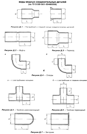
"Виды медных соединительных деталей (по ТУ 5130-001-05480358)"
