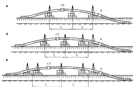
Рисунок 21 — Совмещенный способ изоляции и укладки газопровода диаметром: а — 500–800 мм; б — 800–1000 мм; в — св. 1000 мм при использовании комбайна
