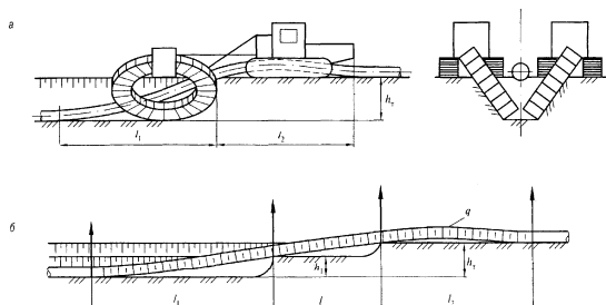
Рисунок 23 — Укладка газопровода методом «подкопа»
