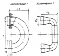
Рис. 3 Калач соединительный
