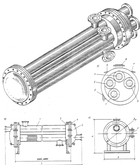
Рис. 5 Общий вид горизонтального многоходового кожухотрубного водоподогревателя
