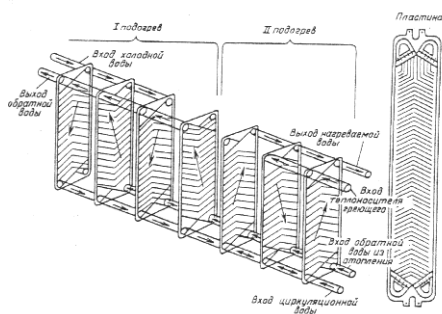
Рис. 3. Схема компоновки водоподогревателей 2 и 22 подогрева в одну установку с противоточным движением воды
