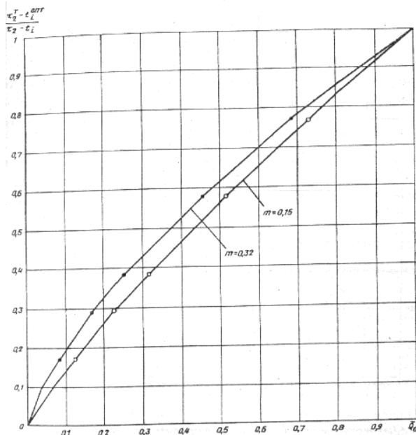
Рис. 3. Графики изменения температурного критерия системы отопления
