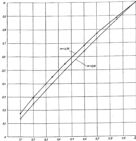
Рис. 4. Графики изменения относительных температур теплоносителя в однотрубных системах отопления при количественно-качественном регулировании
