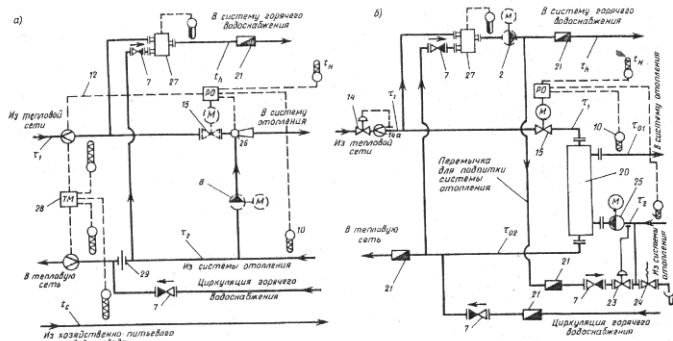
Рис. 9. Схемы присоединения систем горячего водоснабжения и отопления в ИТП при зависимом (а) присоединении системы отопления через элеватор (пунктиром — с циркуляционным насосом) с учетом теплоты по тепломеру и независимом (б) — с учетом теплоты по водомеру
