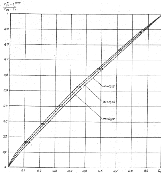
Рис. 2. Графики изменения температурного критерия системы отопления по
