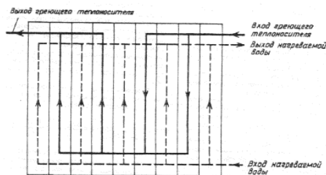
Рис. 2. Несимметричная компоновка пластинчатого водоподогревателя, обозначение Сх (2 + 2)/5
