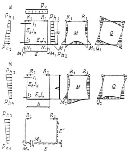
Черт. 4. Расчетная схема тоннеля с шарнирами в уровне плит перекрытия
