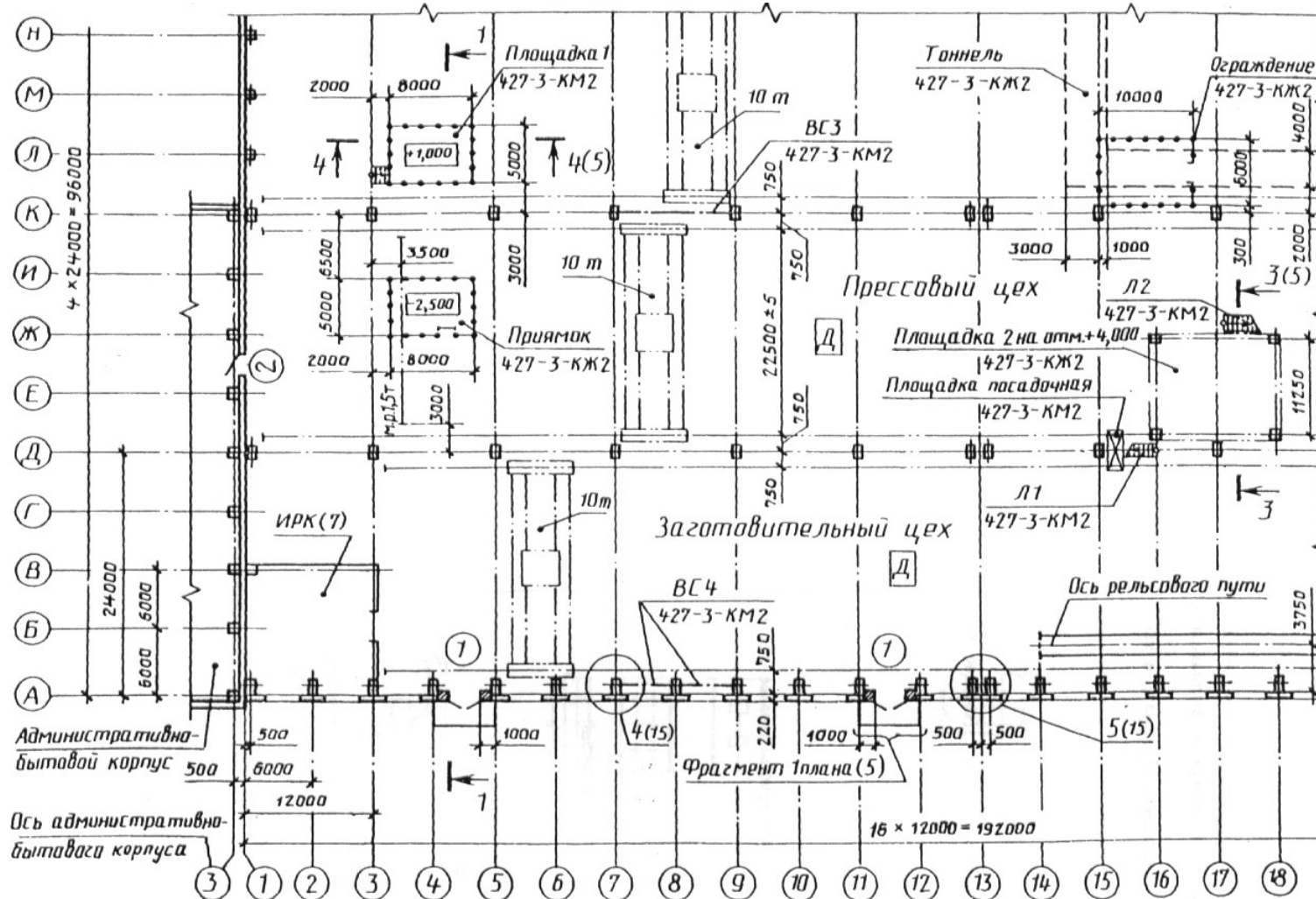
Пример выполнения плана одноэтажного производственного здания
