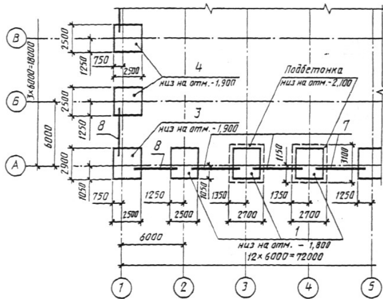
Схема расположения элементов фундаментов и фундаментных балок
