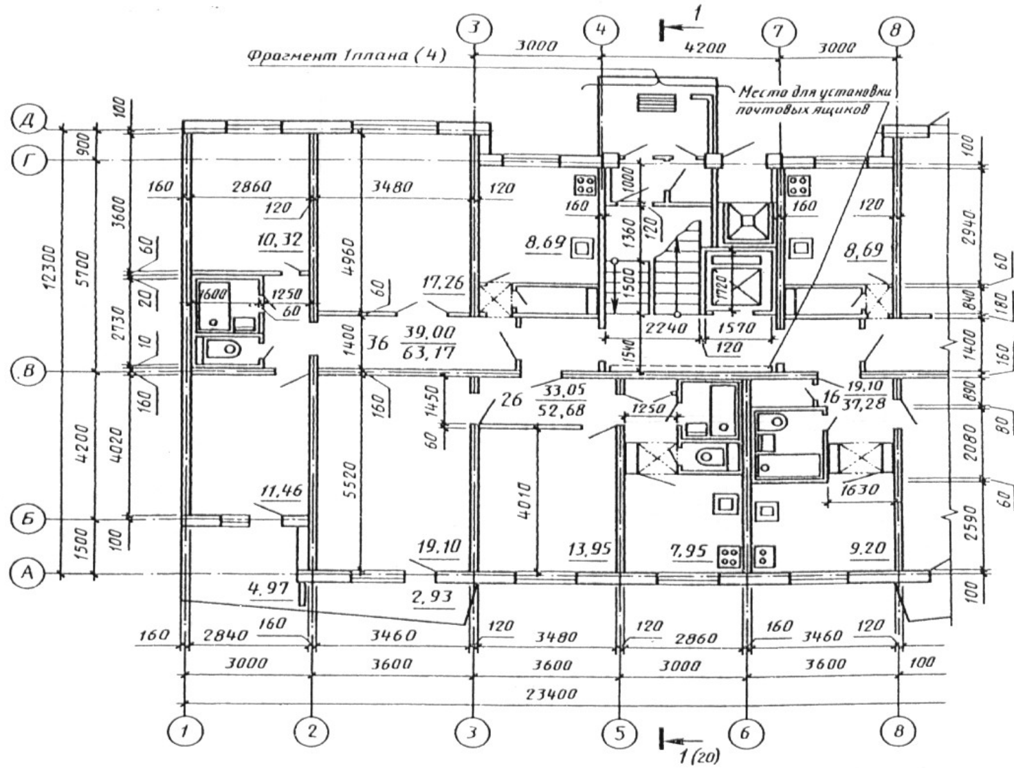
Пример выполнения плана этажа жилого дома
