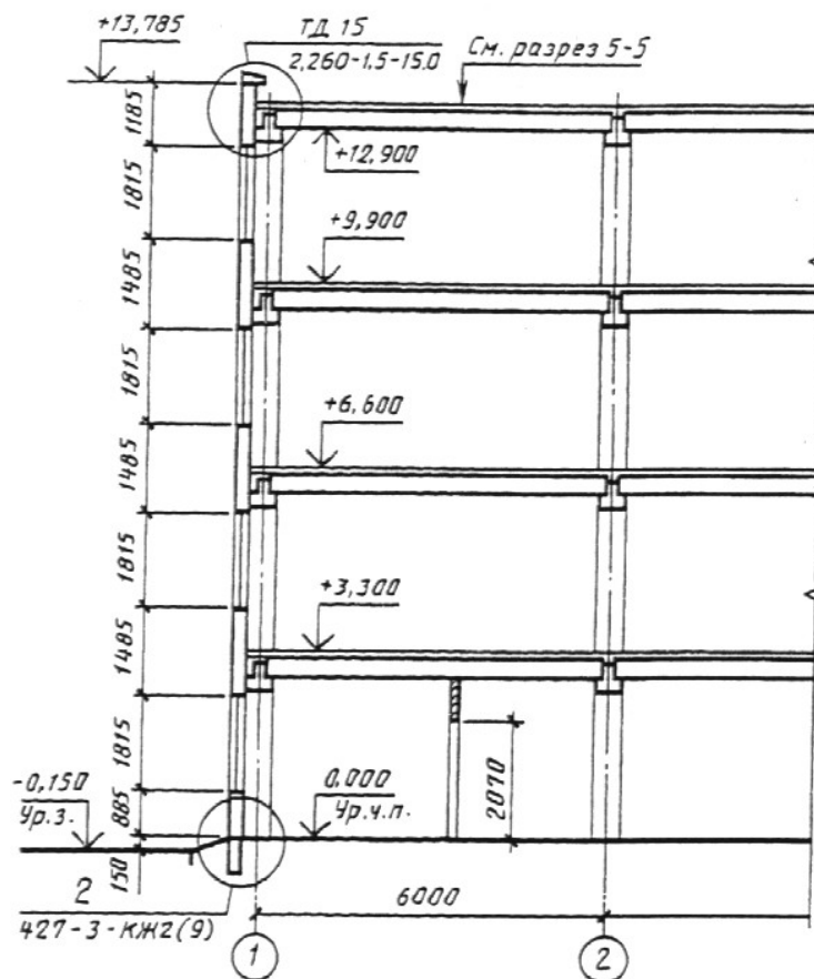
Разрез 2-2
