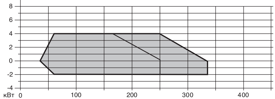
Соотношение регулирования макс. ~ 1 : 10 *
