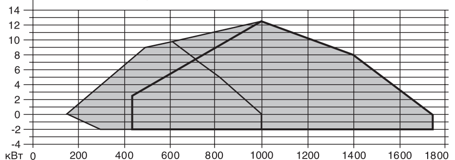
Соотношение регулирования макс. ~ 1 : 10 *
